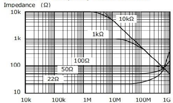
周波数特性 Frequency Characteristics
