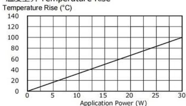
温度上昇 Temperature Rise
