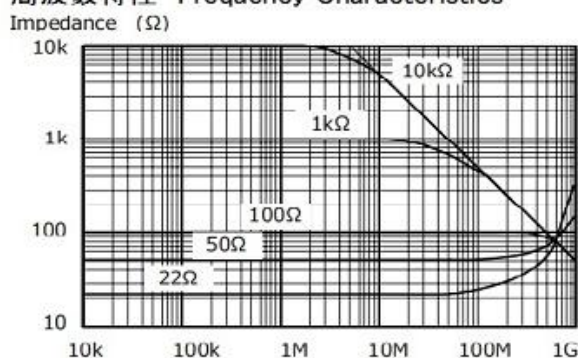
周波数特性 Frequency Characteristics
